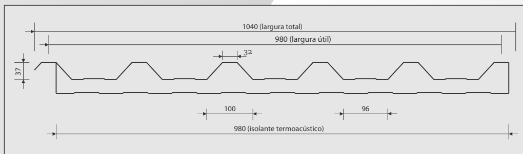
TRAPÉZIO TR 25/1020 - FORRO
