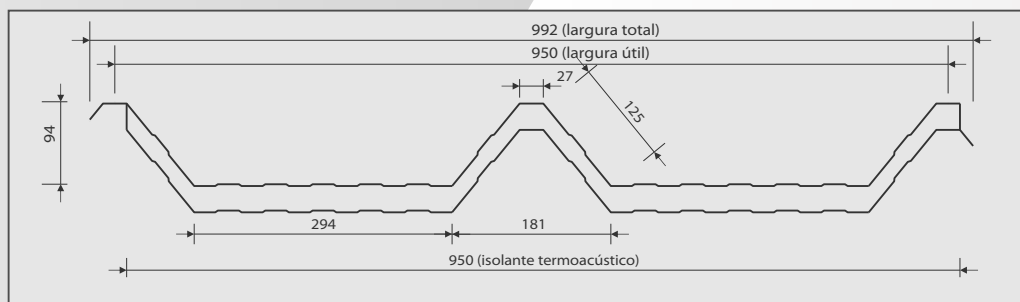
TRAPÉZIO TR 100/950
