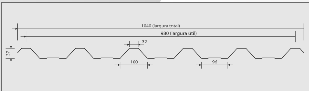
TRAPÉZIO TR 40/980
